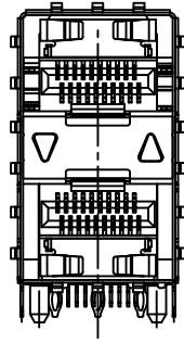
2:Outer Light Pipe
