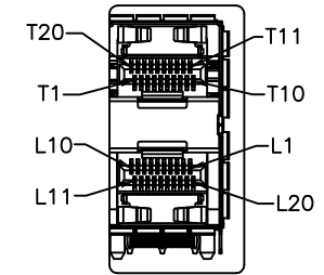
DETAIL A 1:1
