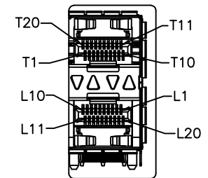
DETAIL A 1:1
