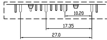
DETAL A
