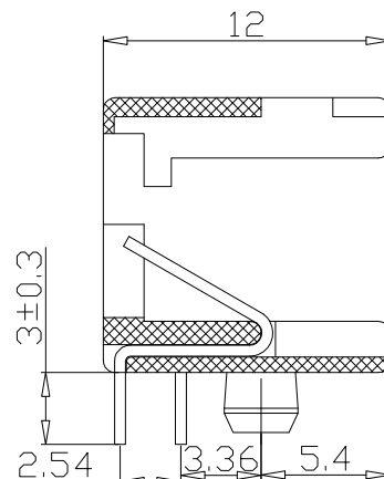
A-A
